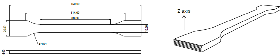
图 1: 拉伸测试样品
